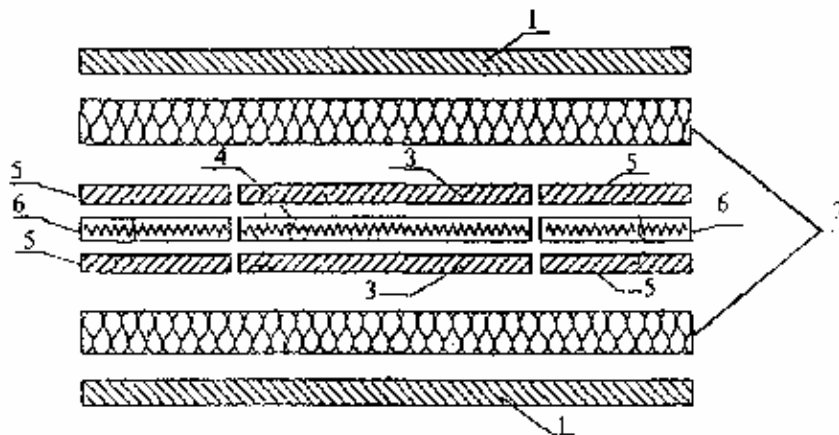
1 — холодильник; 2 — испытываемые образцы; 3 — плиты нагревателя зоны измерения; 4 — обмотка нагревателя зоны измерения; 5 — плиты нагревателя охранной зоны; 6 — обмотка нагревателя охранной зоны
