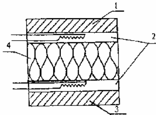
1 — нагреватель; 2 — тепломеры; 3 — холодильник; 4 — испытываемый образец Рисунок А.2 — Схема прибора с двумя тепломерами
