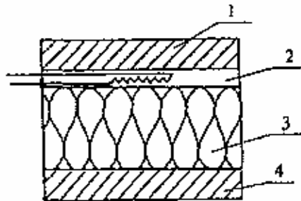
1 — нагреватель; 2 — тепломер; 3 — испытываемый образец; 4 — холодильник Рисунок А.1 — Схема прибора с одним тепломером
